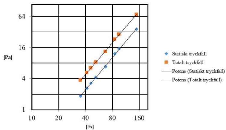
Tryckfallsdiagram vid 45° taklutning
