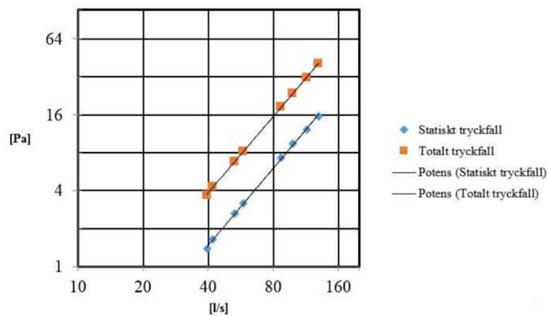
Tryckfallsdiagram vid 14° taklutning
